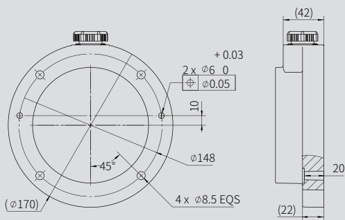
AUBO-D7S 底座俯视图
