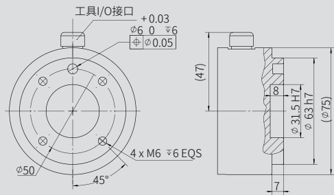
AUBO-D7S 末端法兰
