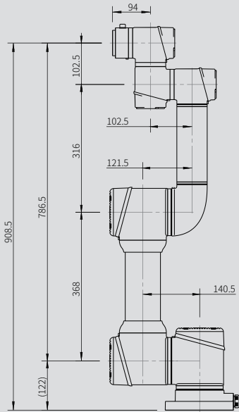
AUBO-D7S 外形尺寸图
