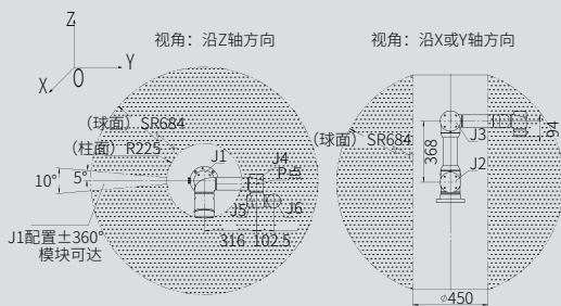
AUBO-D7S 本体P点运动范围
