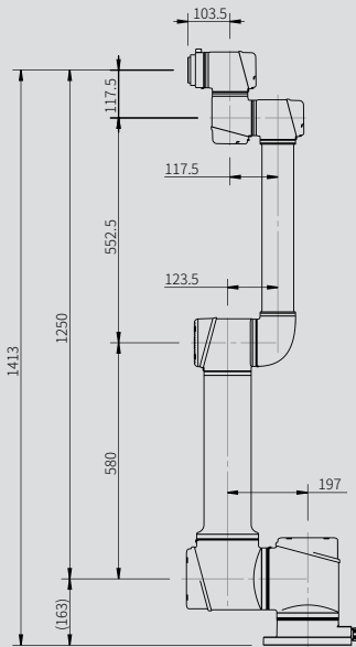
AUBO-D12S 外形尺寸图
