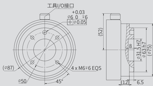
AUBO-D12S 末端法兰
