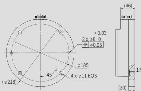
AUBO-D12S 基座俯视图
