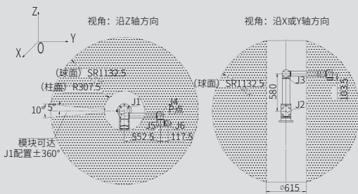
AUBO-D12S 本体P点运动范围
