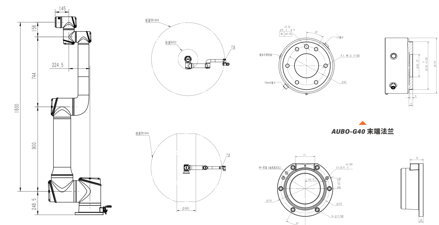
AUBO-G40 外形尺寸图
