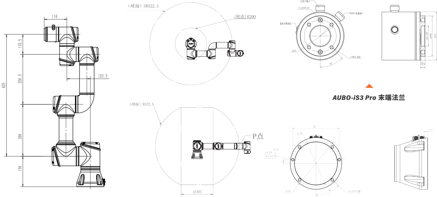
AUBO-iS3 Pro 外形尺寸图
