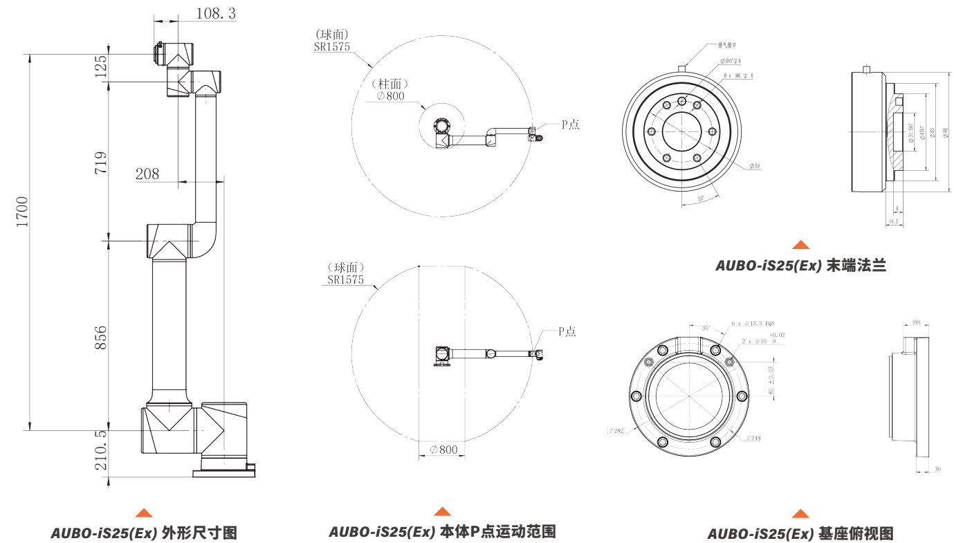
iS25(Ex) 尺寸图
