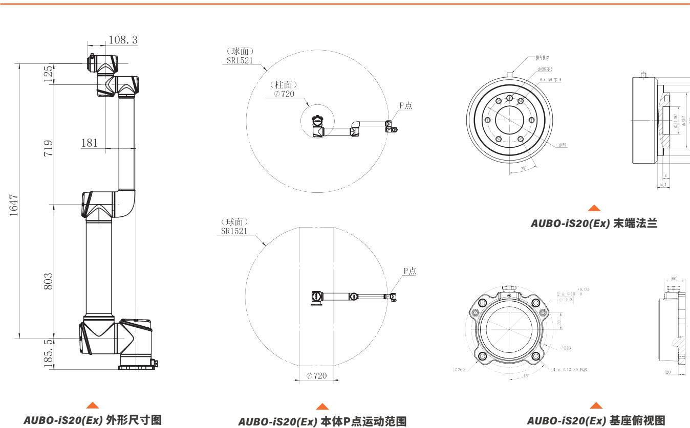
iS20(Ex) 尺寸图
