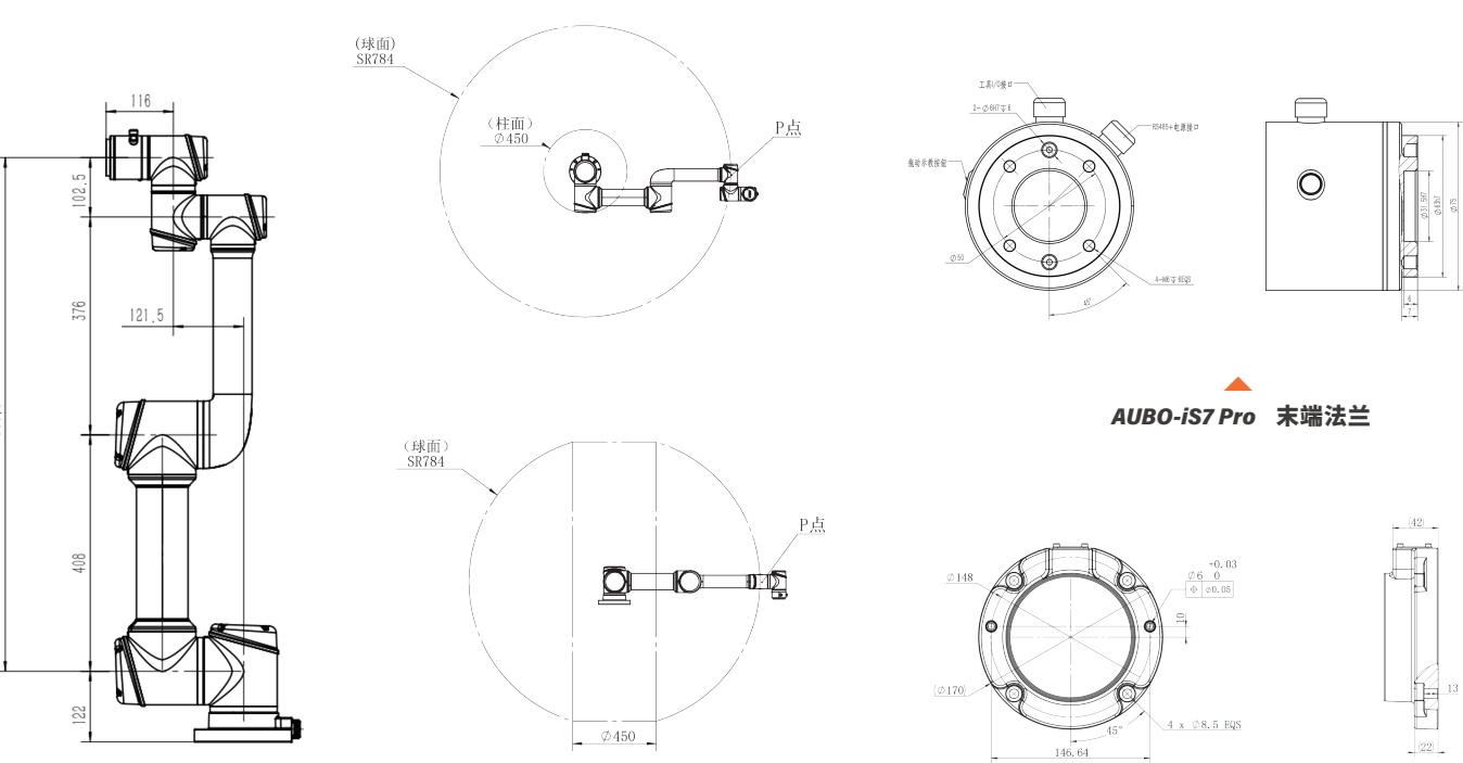
AUBO-iS7 Pro 外形尺寸图
