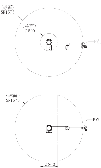
AUBO-iS25 本体P点运动范围
