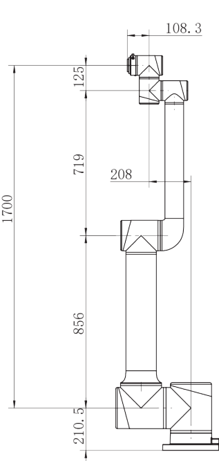
AUBO-iS25 外形尺寸图
