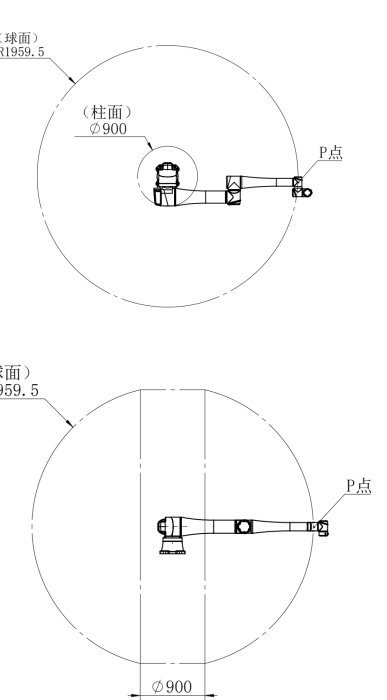
AUBO-iS35 本体P点运动范围
