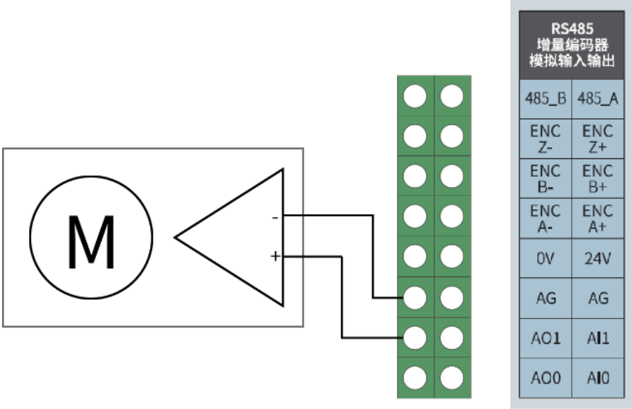
图 7-10 模拟电压输出连接驱动设备接线示意图
