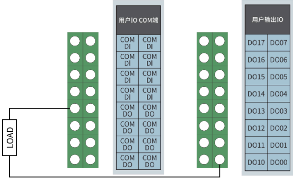
图 7-7 数字输出接口连接负载示意图
