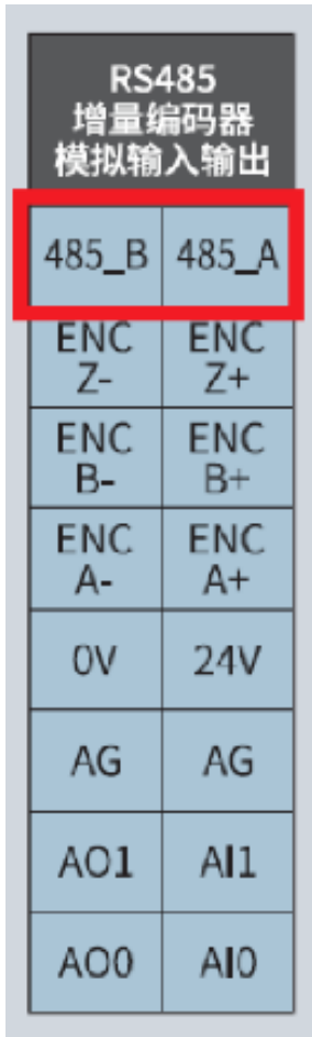
图 7-11 端子排 RS485 接口示意图
