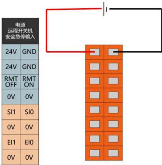
图 7-5 外部电源供电示意图
