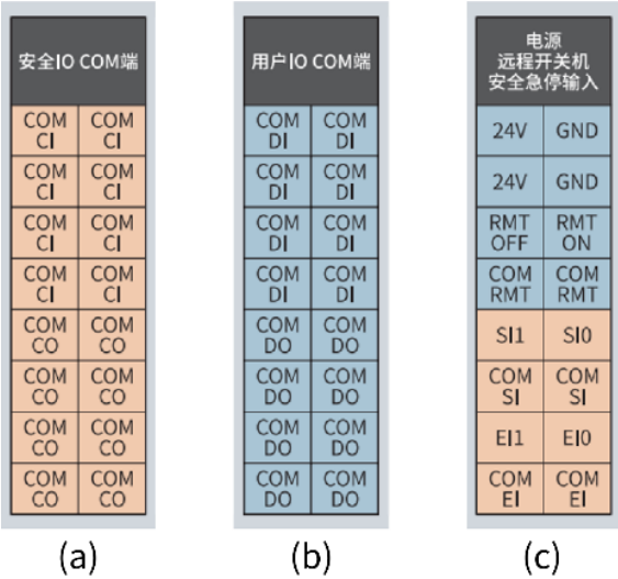
图 7-3 公共 COM 端示意图
