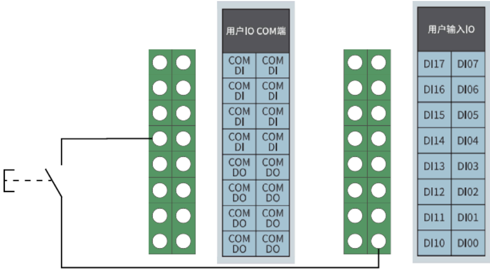
图 7-6 数字输入接口连接按钮开关示意图
