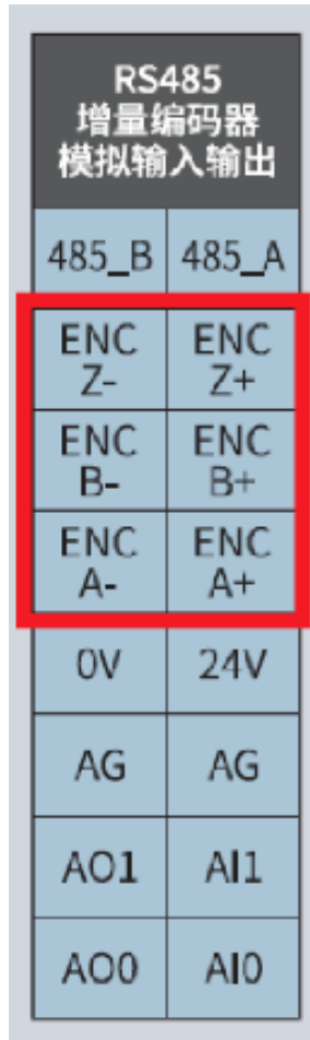
图 7-12 增量编码器接口示意图
