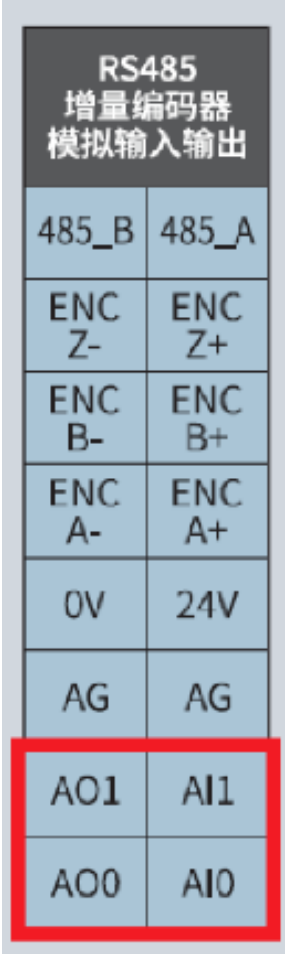
图 7-8 模拟 I/O 接口示意图
