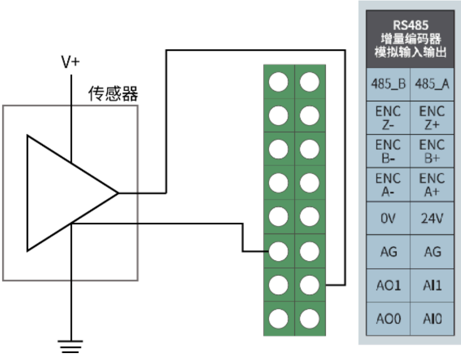
图 7-9 模拟电压输入连接传感器接线示意图
