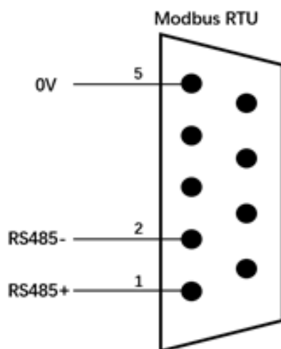
图 7-1 RS485 接口引脚说明图
