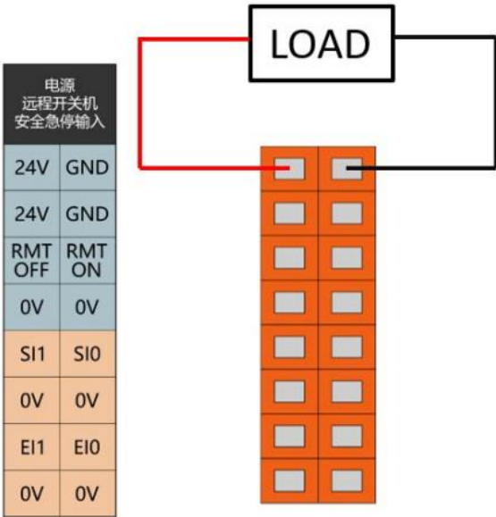
图 7-4 内部电源供电示意图
